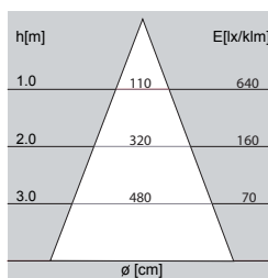
1100 Lumens 4000K 60°
